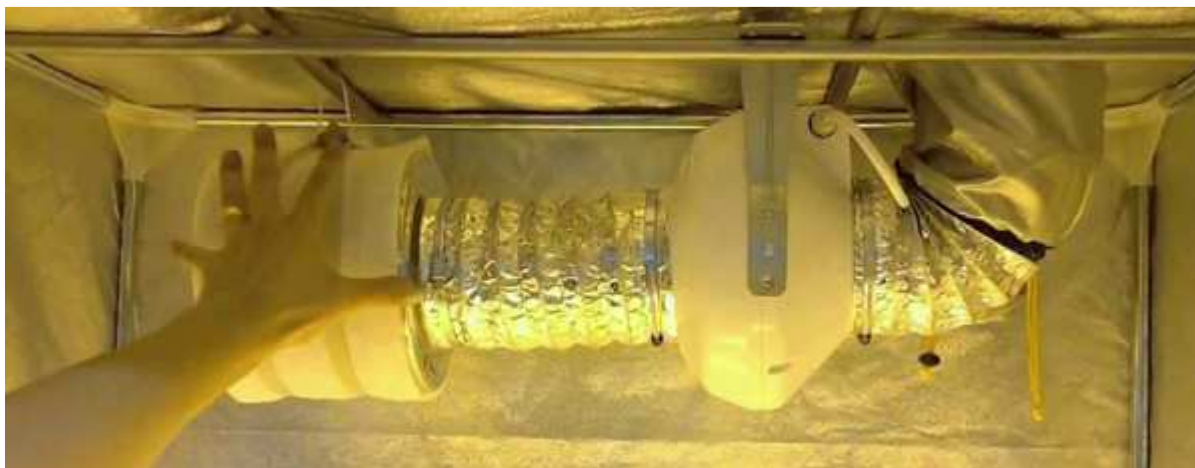
Ejemplo conexión extractor vk 150 dentro del armario con filtro
